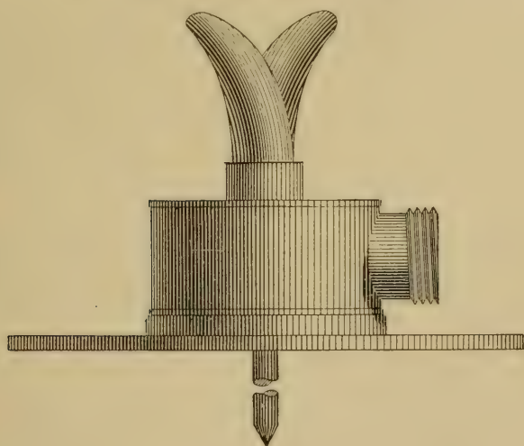
FIG. 6.—Nozzle.
